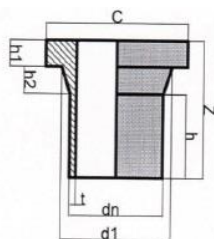
فلنج TAPE B پلی اتیلن مطابق استاندارد ISIRI 14427/PE100
